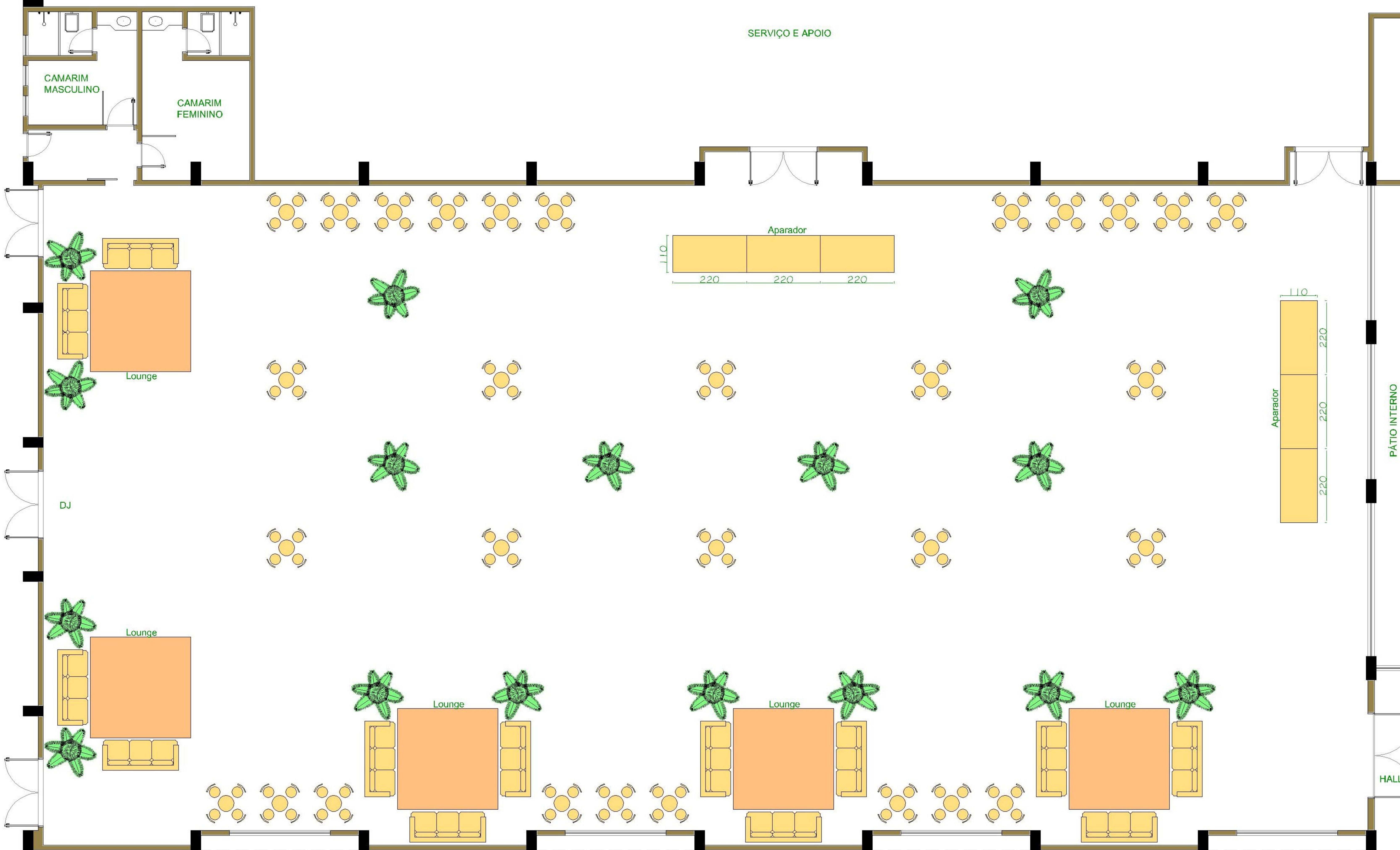
PLANTA BAIXA - SALÃO PRINCIPAL
